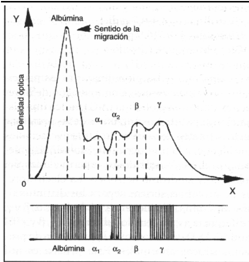
FIGURA 12-1. Electroforograma normal.
